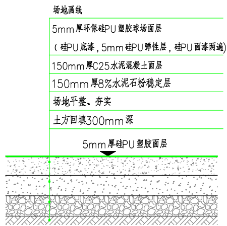
5mm厚硅PU球场剖面图
